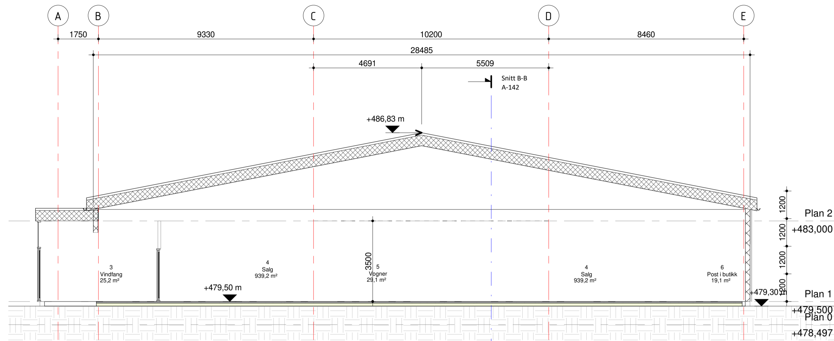
Snitt A-A - Inngang 1 : 100
